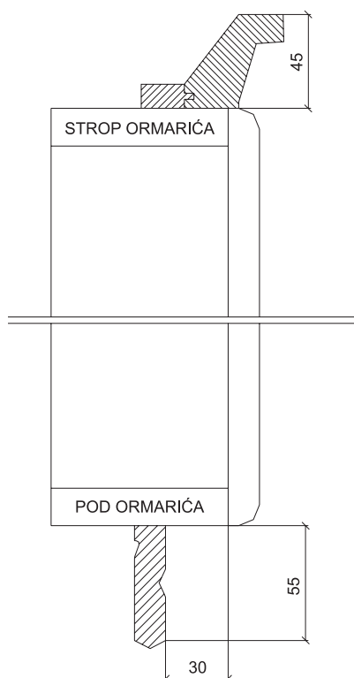
PRIKAZ POSTAVLJANJA GUL-a I DUL-a
